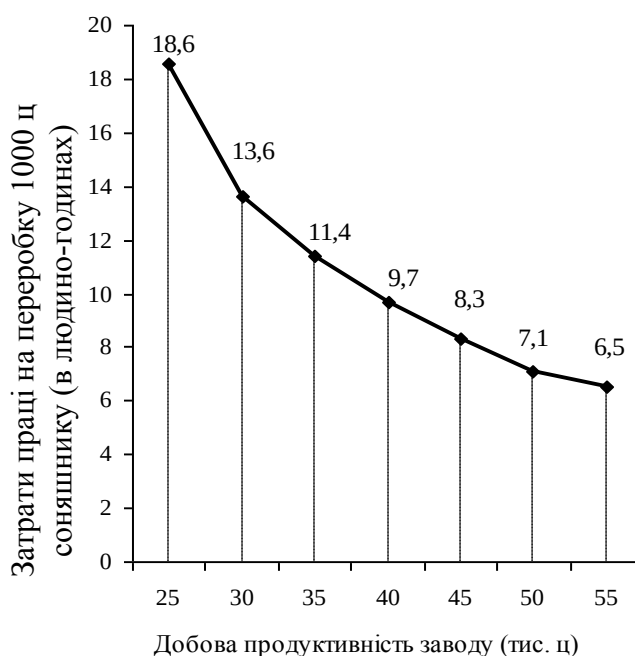
Рис. 5.1. Залежність затрат робочого часу на переробку 1000 ц соняшнику від розмірів фактичного добового випуску на олійних заводах.
