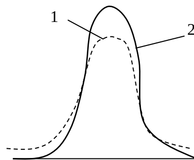
Рис. 12.1. 1 — крива розподілу Стюдента; 2 — крива нормального розподілу.
