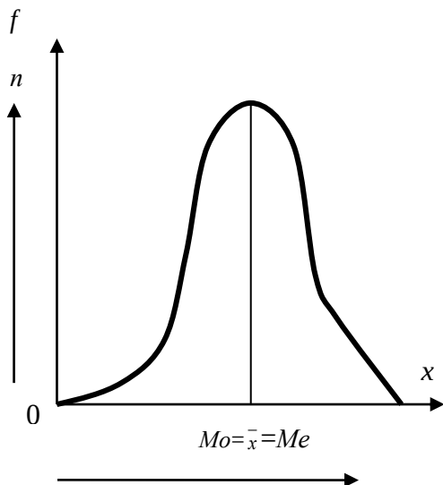
Рис. 8.12. Симетричний нормальний розподіл.
